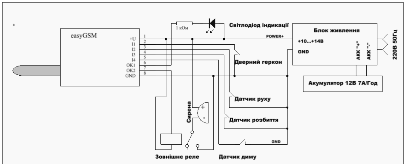
Малюнок 8. Приклад підключення easyGSM у якості 4-х зонної охоронної сигналізації без використання зовнішньої клавіатури-шифратора.
