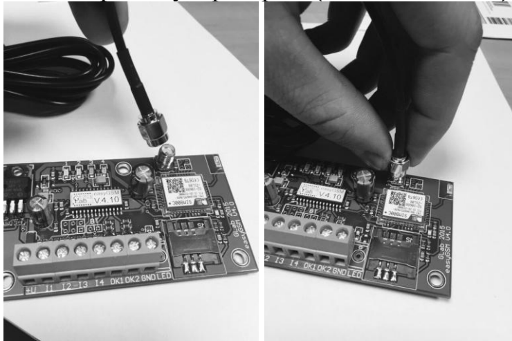
Малюнок 2. Підключення антени.
