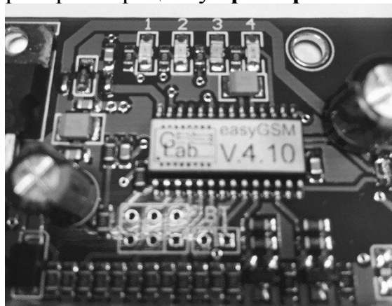
Малюнок 4. Світлодіоди індикації.
