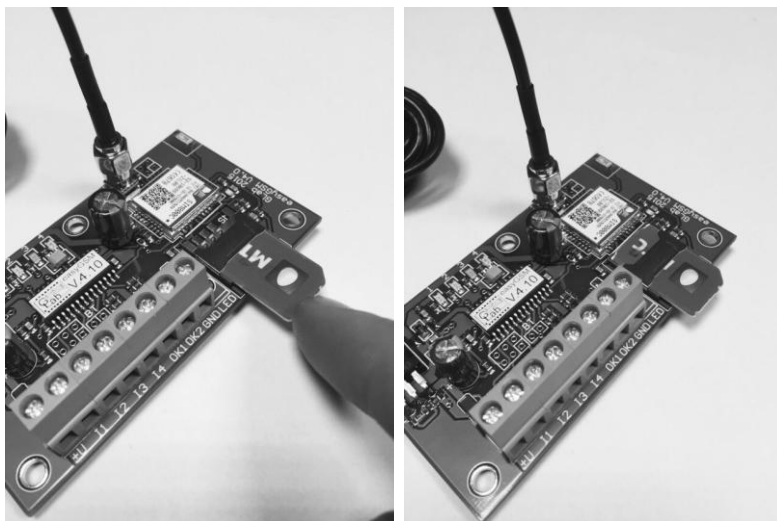
Малюнок 3. Встановлення SIM карти.
