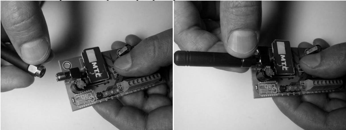
Малюнок 2. Підключення антени.
