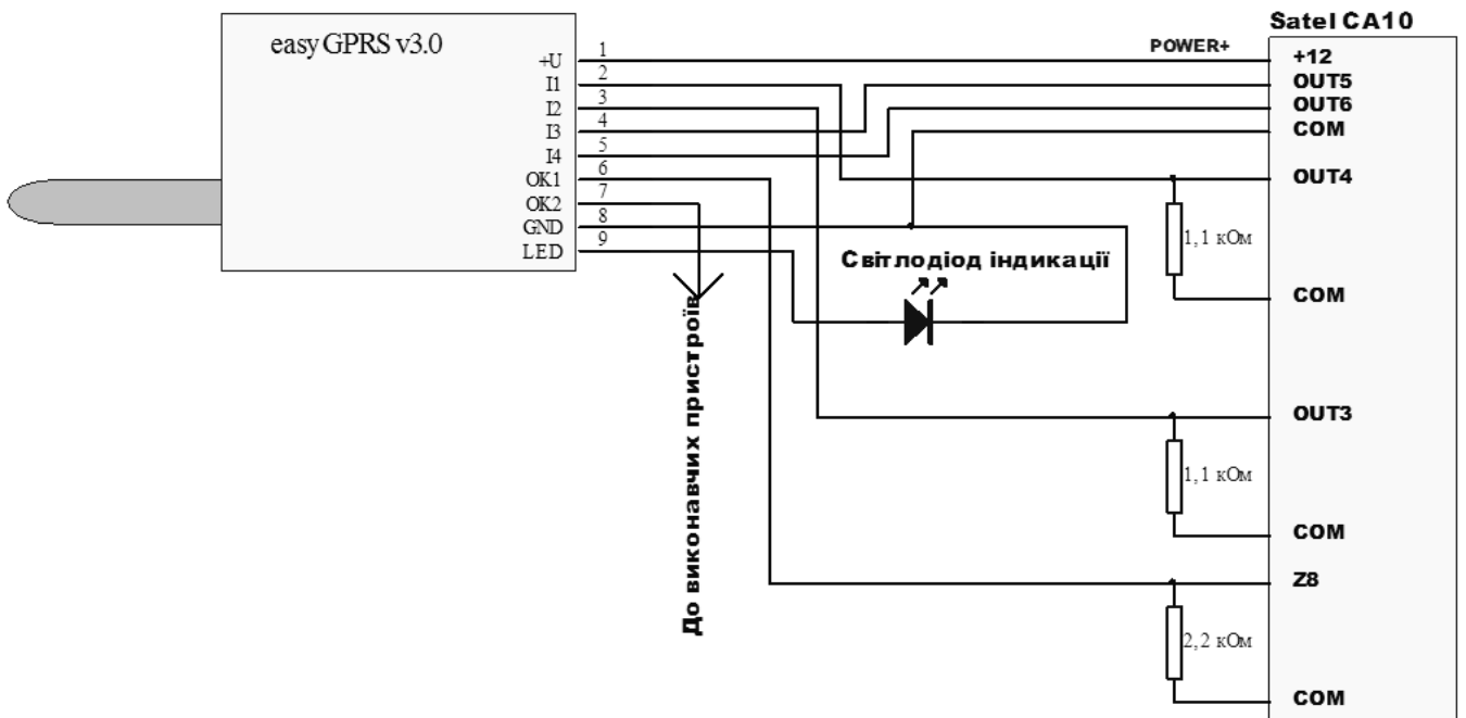
Малюнок 6 Приклад підключення easyGPRS до Satel CA10.
