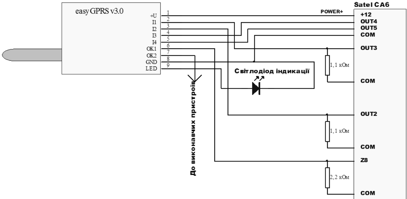
Малюнок 5. Приклад підключення easyGPRS до Satel CA6.
